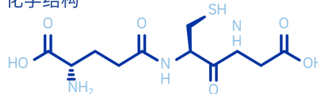
化学结构
